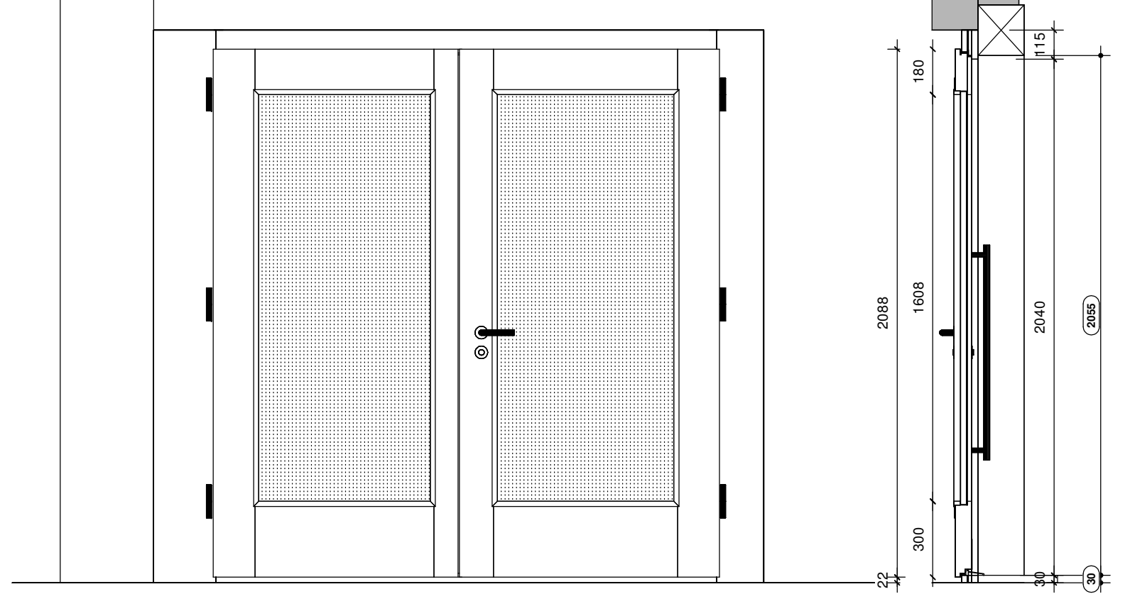
Ansicht Aussen
